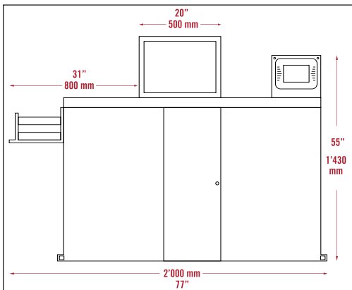
Vorderansicht
