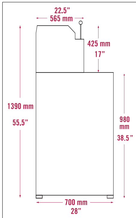
Seitenansicht
