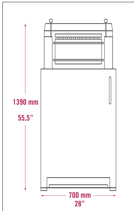
Abmessungen: Vorderansicht
