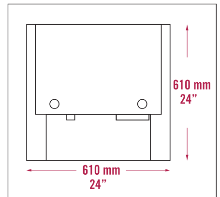
Grundriss
