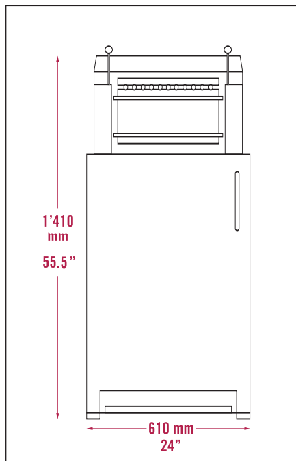
Abmessungen: Vorderansicht
