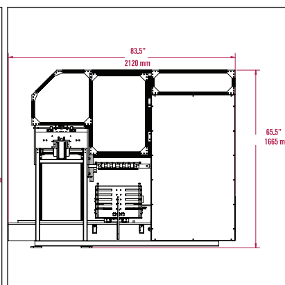
Hotmelt-Auftragsgerät Nordson (Option) zur Verstärkung der Scharnierzone und die Kaltleimpumpe (PVA) mit elektronischer Steuerung für einen präzisen Düsenauftrag.
