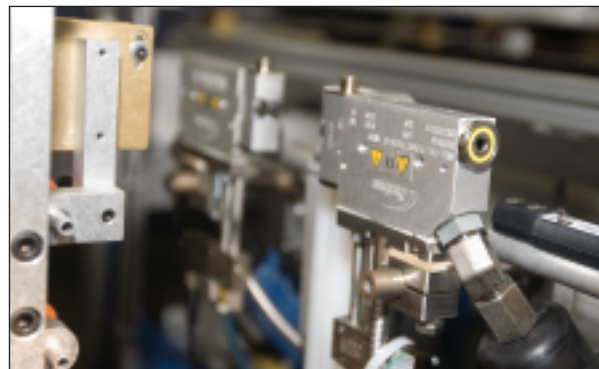
Hotmelt-Auftragsgerät Nordson (Option) zur Verstärkung der Scharnierzone und die Kaltleimpumpe (PVA) mit elektronischer Steuerung für einen präzisen Düsenauftrag.
